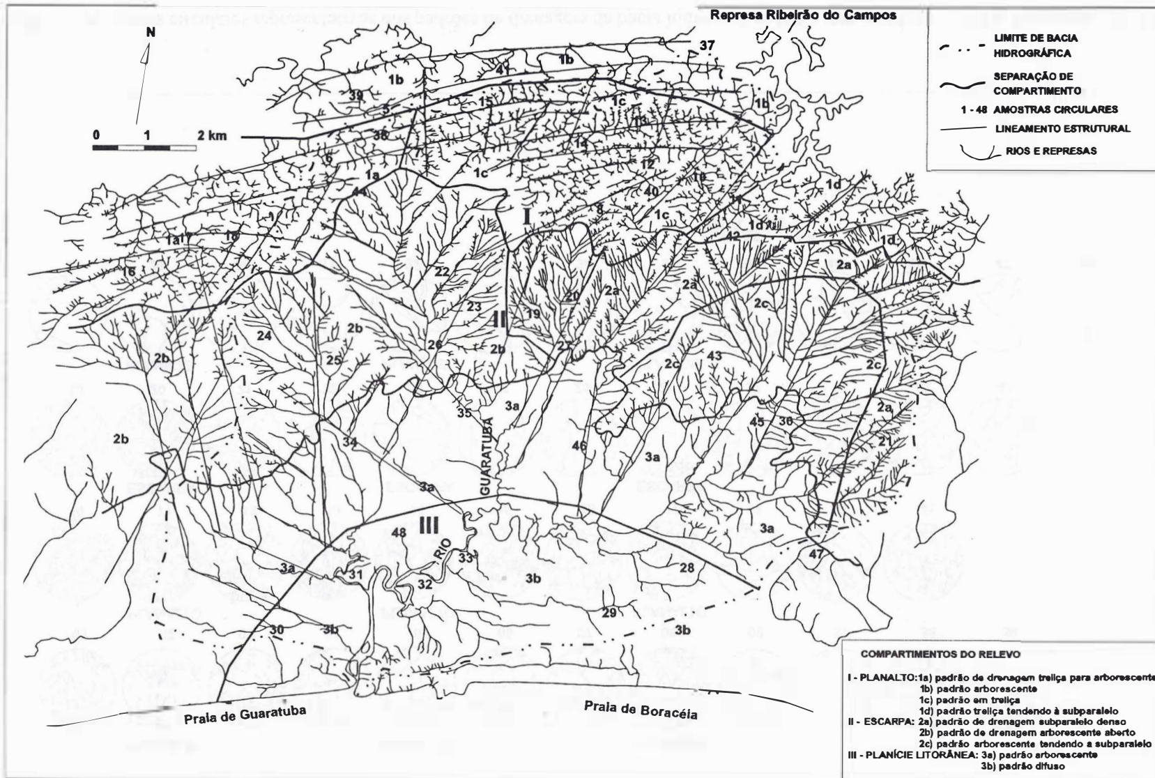
FIGURA 2 - Mapa detalhado da rede de drenagem da bacia hidrográfica do Guaratuba, com indicação da posição das amostras circulares.
