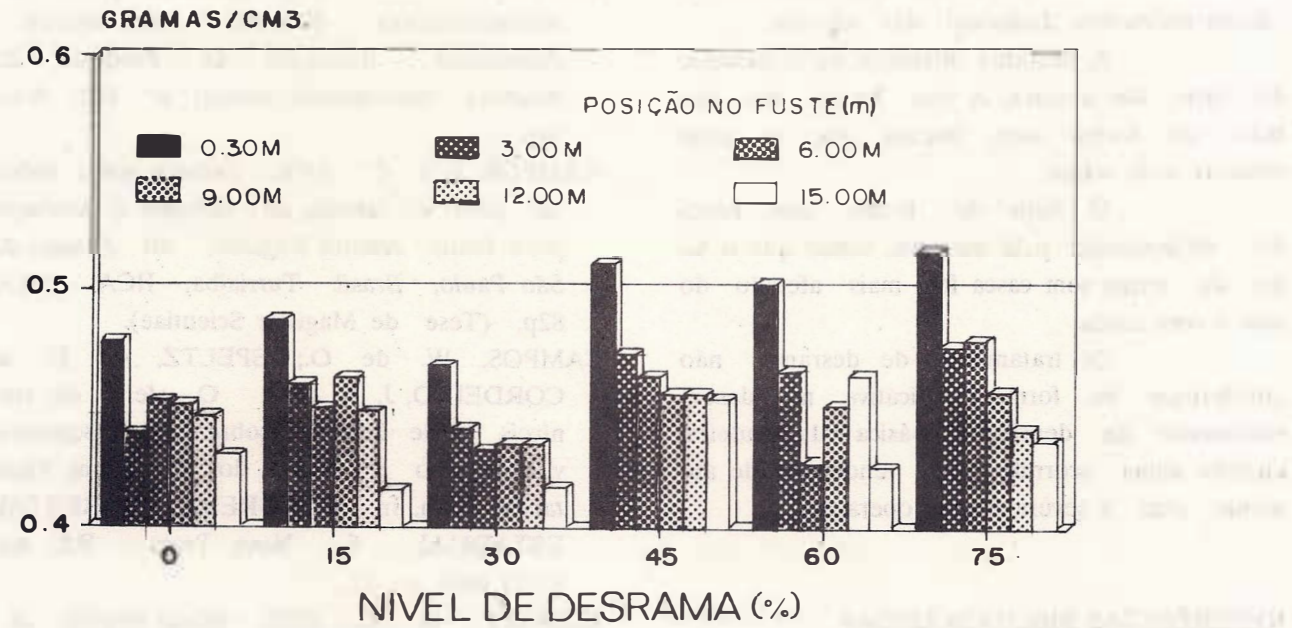
FIGURA 5 -Variação da densidade básica da madeira em função da desrama e posição no fuste.
