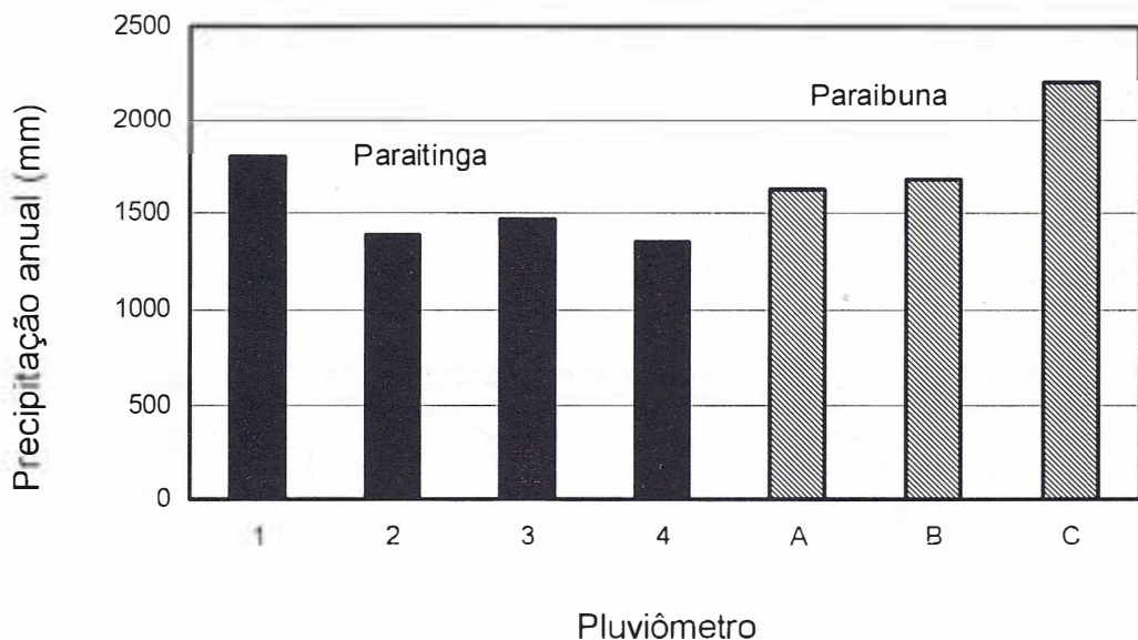
FIGURA 2 - Médias anuais de precipitação nas bacias dos rios Paraibuna e Paraitinga.
