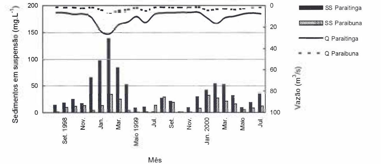
FIGURA 4 - Variação da concentração de sedimentos em suspensão (SS) e da vazão instantânea (Q) dos rios Paraibuna e Paraitinga.
